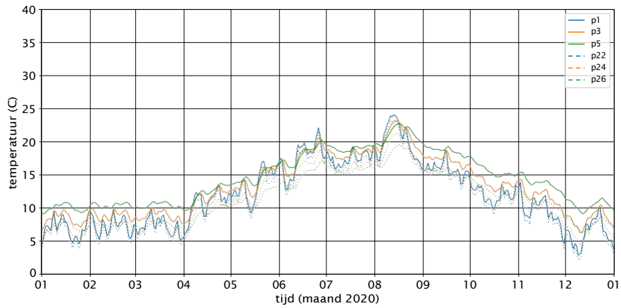
Figuur 4.15 Temperatuurverloop rekenpunten profiel 8.
