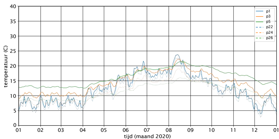
Figuur 4.8 Temperatuurverloop rekenpunten profiel 4.
